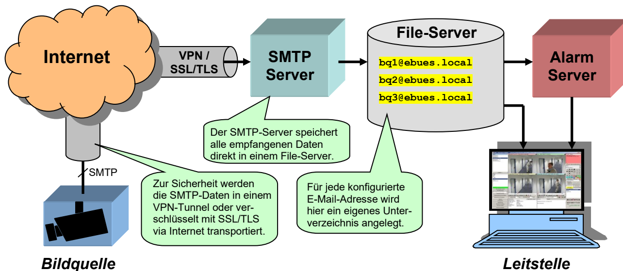
Abbildung 2: AccAlarmReceiverSmtip als SMTP-Server mit AlarmServer und EBÜS Arbeitsplätzen
