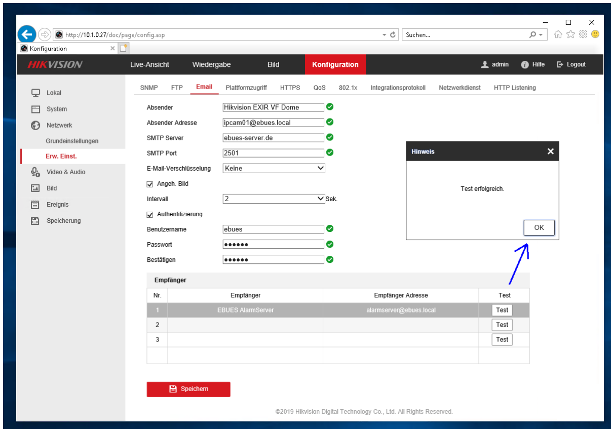
Abbildung 18: Konfiguration von Hikvision-Bildquellen für den Versand von E-Mails
