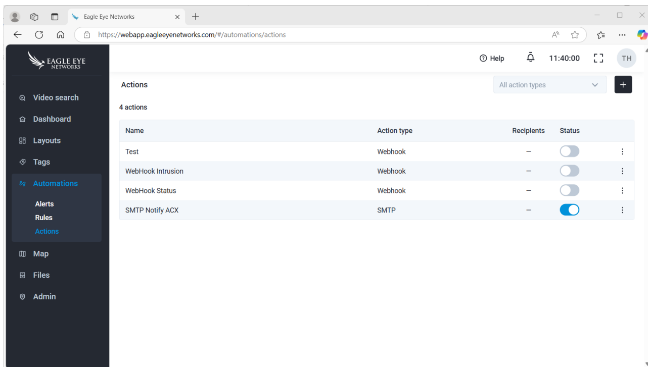
Abbildung 43: Konfiguration der EEN Plattform für den Versand von SMTP-Nachrichten
