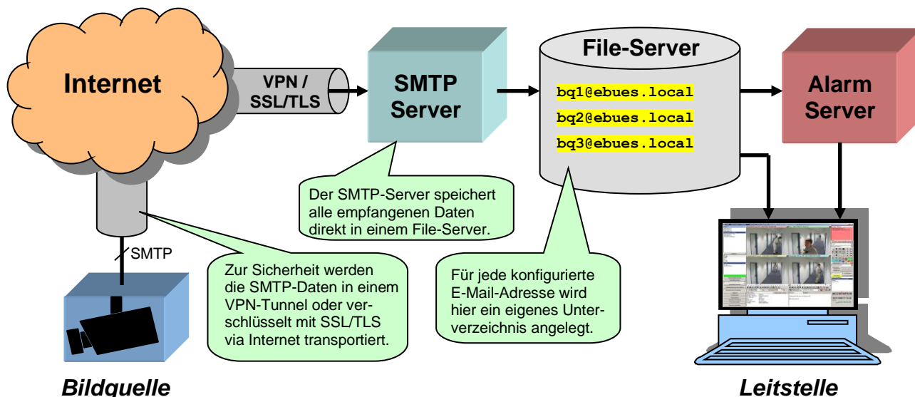
Abbildung 2: AccAlarmReceiverSmtP als SMTP-Server mit AlarmServer und EBÜS Arbeitsplätzen
