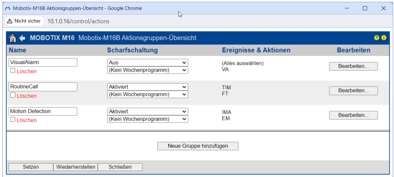
Abbildung 41: Übersicht der Aktionsgruppen
