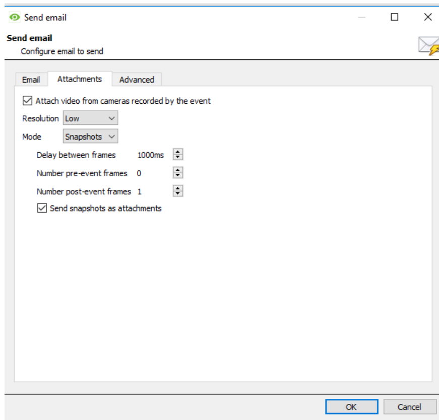
Abbildung 16: Konfiguration von Cathexis-Bildquellen für den Versand von E-Mails (Schritt 4)
