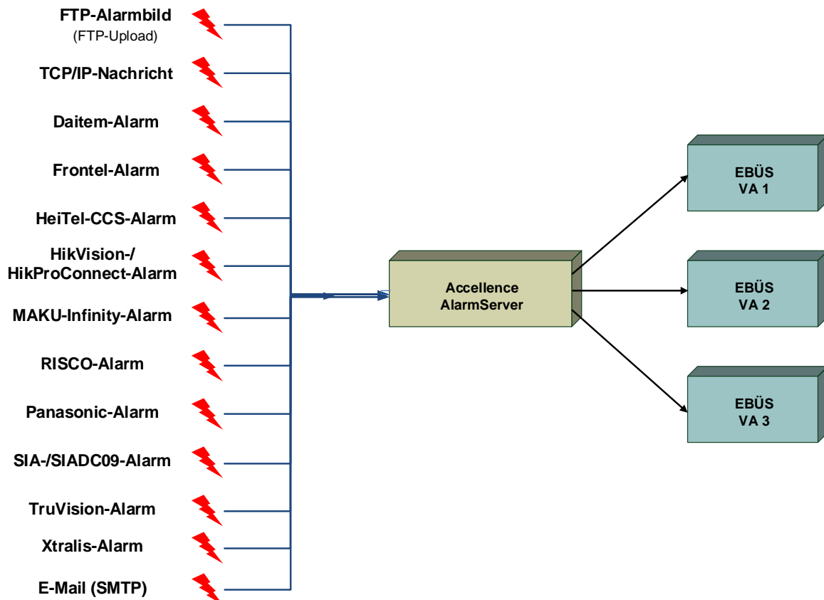
Abbildung 1: Accellence Alarm Server mit EBÜS Video-Arbeitsplätzen (VA)
