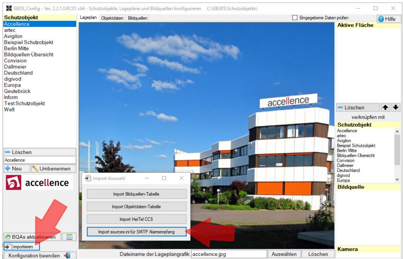
Abbildung 8: Buttons für den Import der Datei sources . ini in EBÜS-Config
