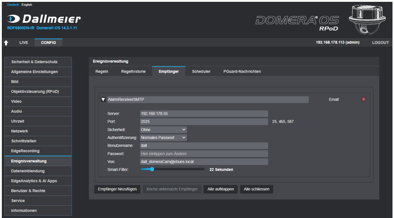
Abbildung 23: Domera-Kamera: Konfiguration eines Empfängers für SMTP-Nachrichten
