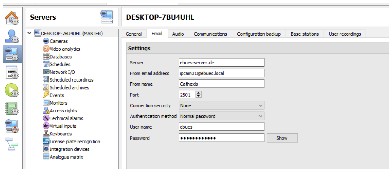
Abbildung 13: Konfiguration von Cathexis-Bildquellen für den Versand von E-Mails (Schritt 1)
