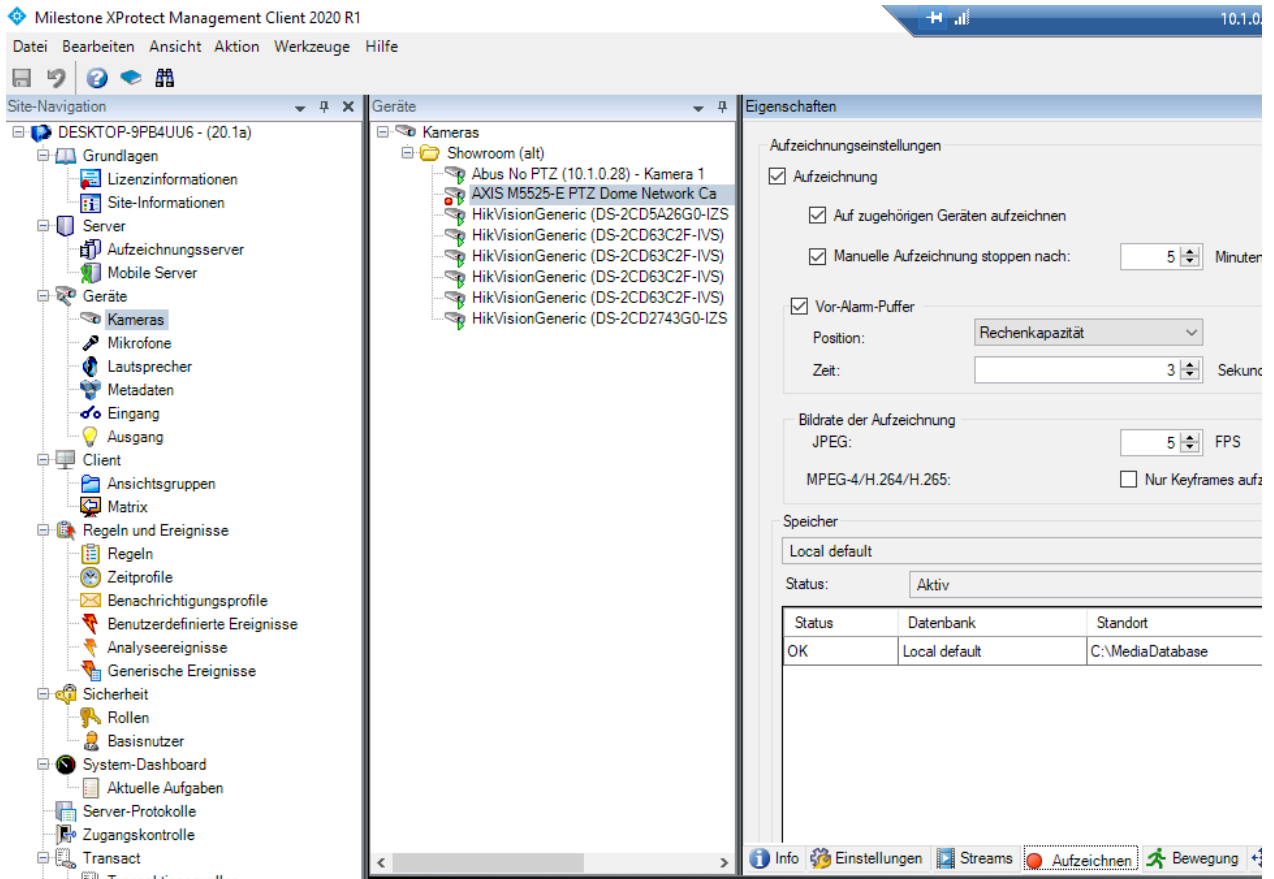
Abbildung 36: Konfiguration von Milestone-Bildquellen für den Versand von E-Mails (Schritt 9)
