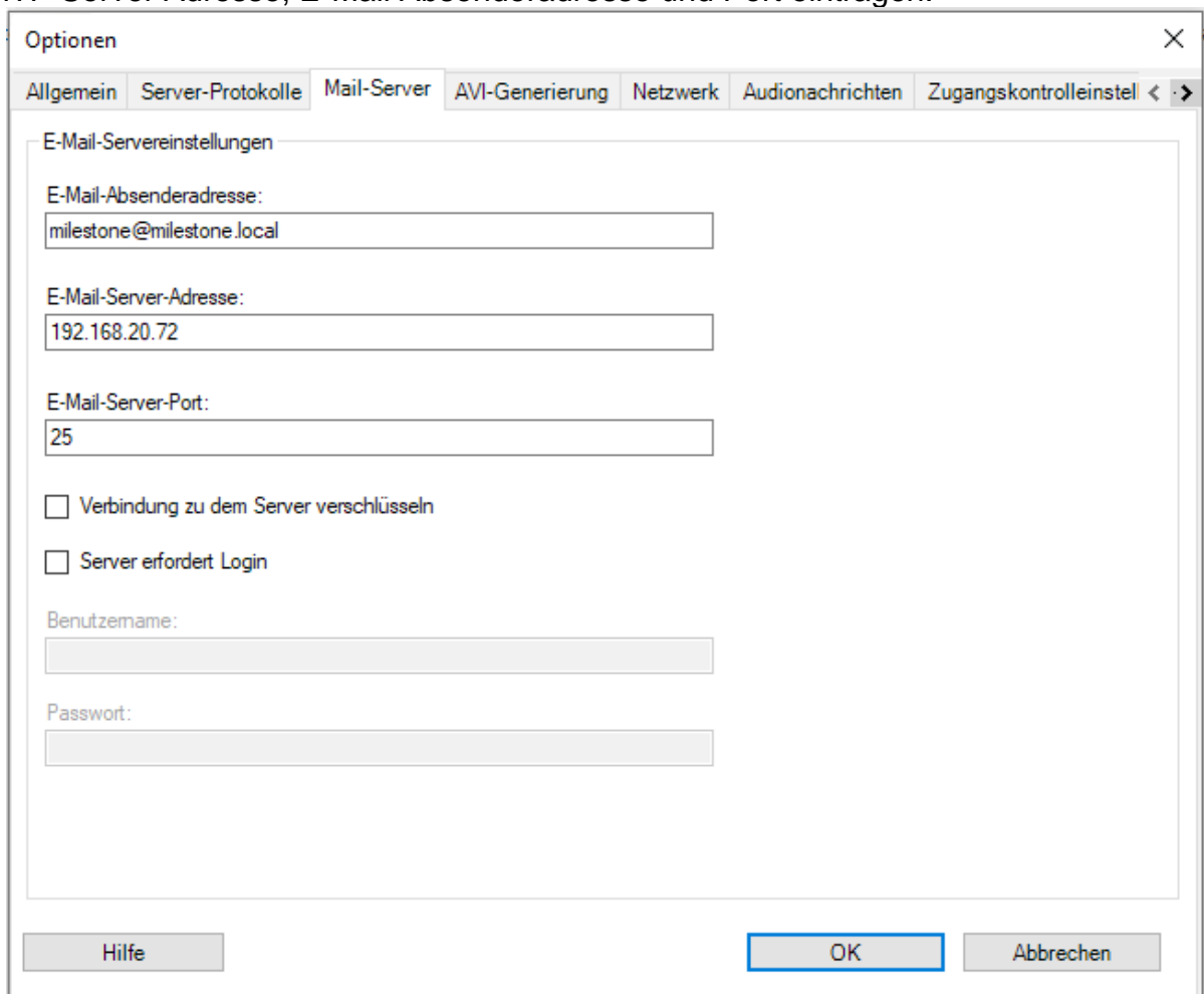
Abbildung 29: Konfiguration von Milestone-Bildquellen für den Versand von E-Mails (Schritt 2)
