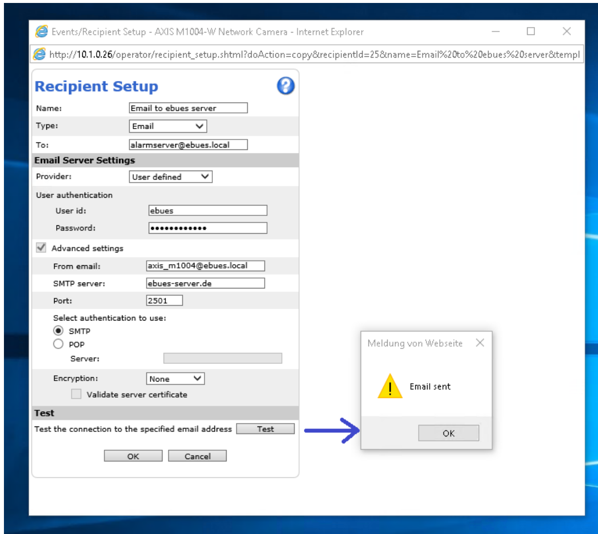
Abbildung 11: Konfiguration von AXIS-Bildquellen für den Versand von E-Mails
