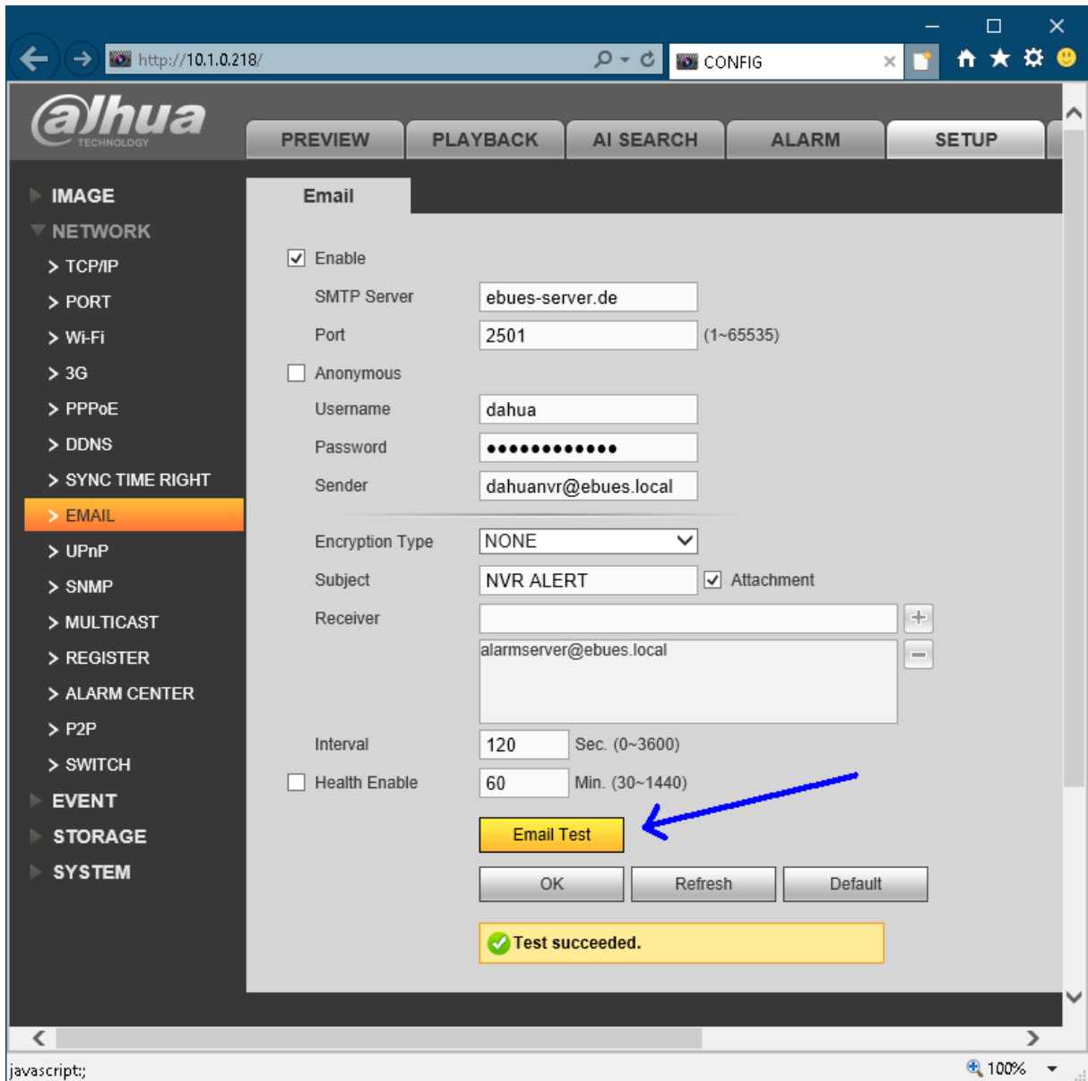
Abbildung 17: Konfiguration von Dahua-Bildquellen für den Versand von E-Mails
