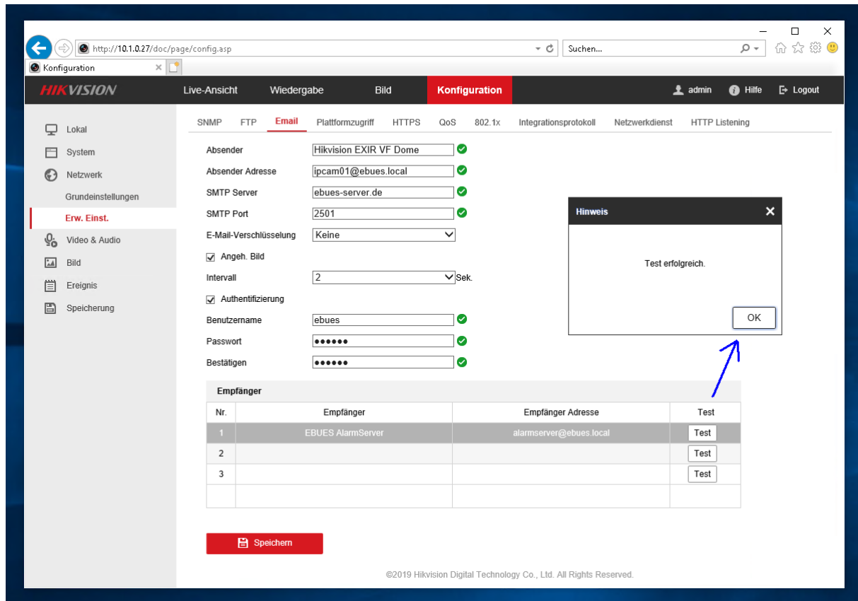
Abbildung 25: Konfiguration von Hikvision-Bildquellen für den Versand von E-Mails
