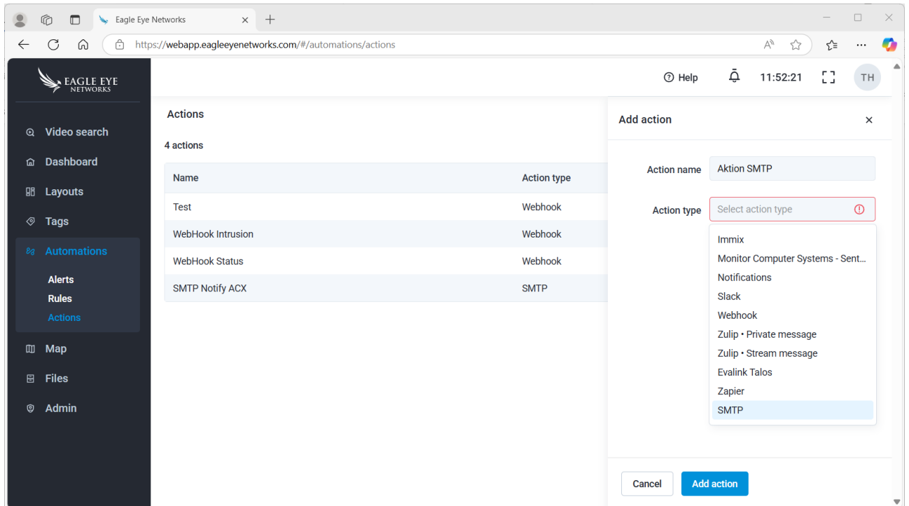
Abbildung 44: Anlegen einer neuen 'Aktion'
