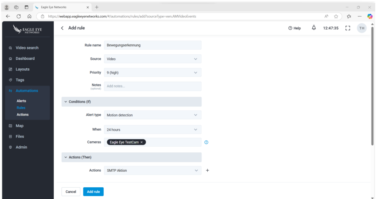
Abbildung 47: Anlegen von Regeln
