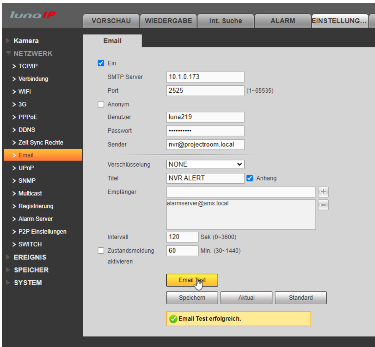
Abbildung 26: Konfiguration von LunaIP-Bildquellen für den Versand von E-Mails
