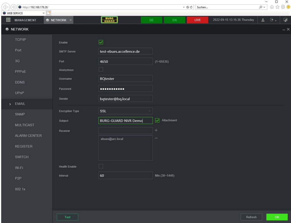
Abbildung 12: Konfiguration von BURG GUARD-Bildquellen für den Versand von E-Mails
