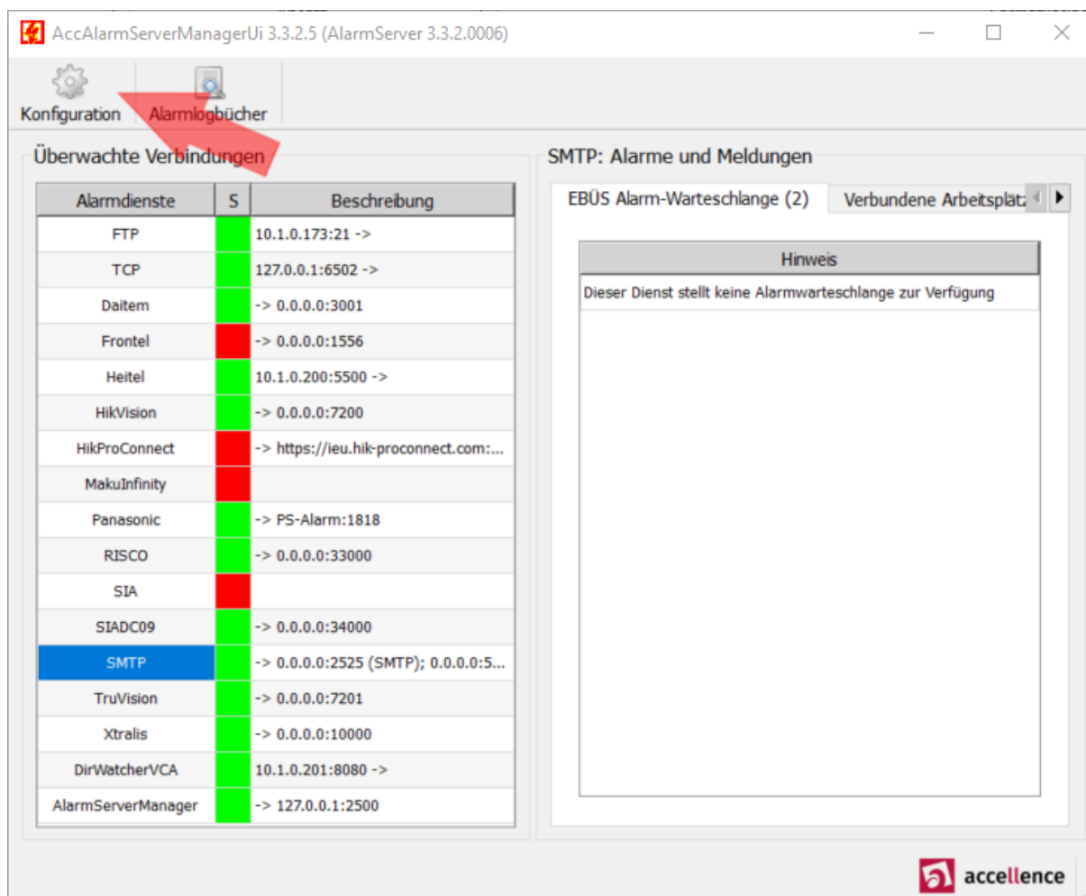
Abbildung 3: AccAlarmServerManagerUI
