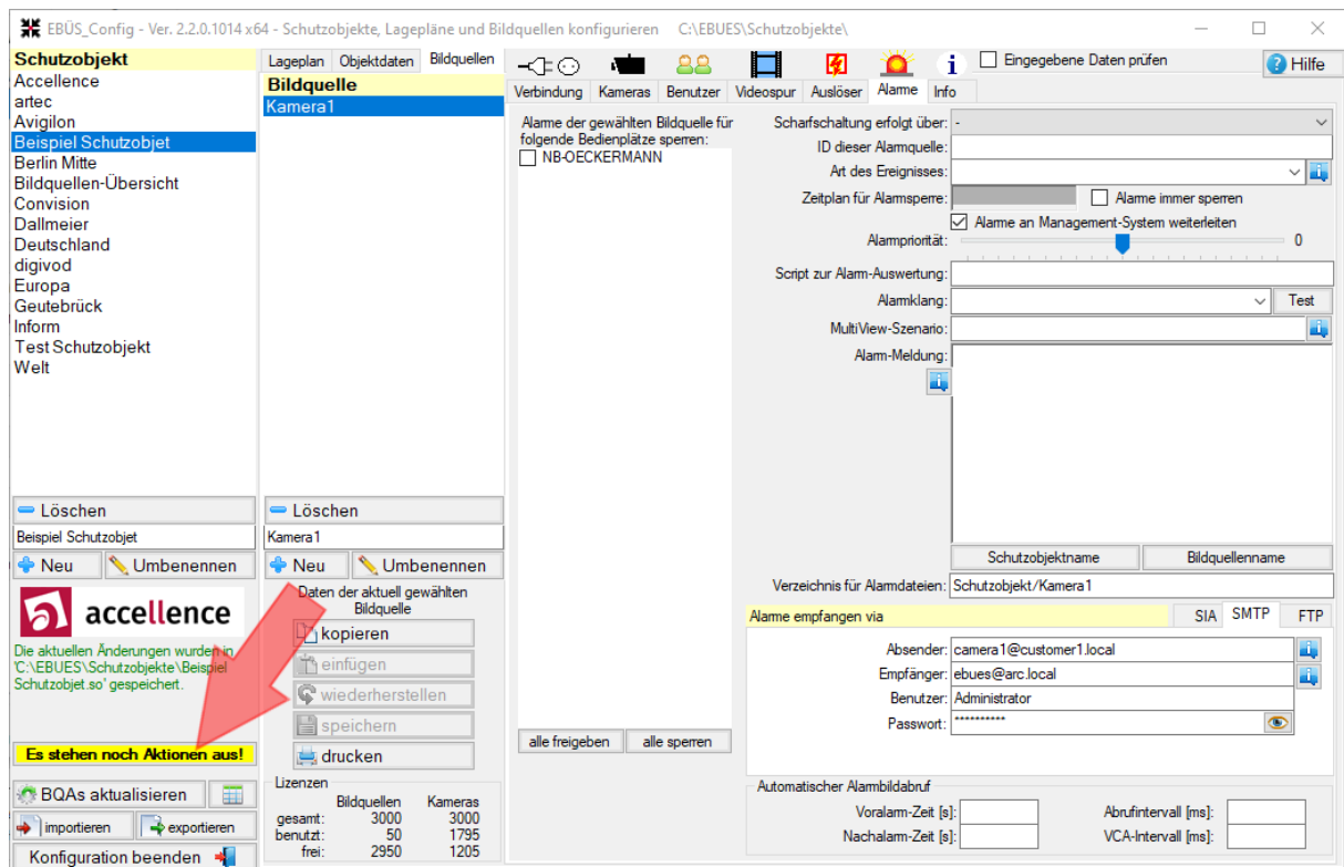
Abbildung 6: Beispiel für gespeicherte SMTP-Einstellungen mit anschließender Warnung
