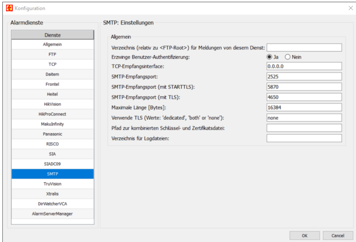
Abbildung 4: Beispiel für Konfiguration des AccAlarmReceiverSMTP (Dienst „SMTP“) in der AccAlarmServerManagerUI
