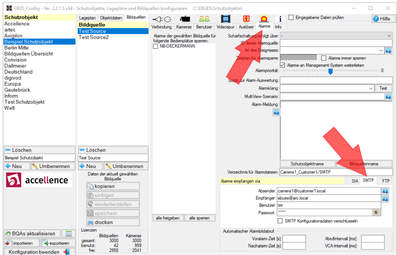
Abbildung 5: Beispiel für Konfiguration für den Alarm Empfang via SMTP
