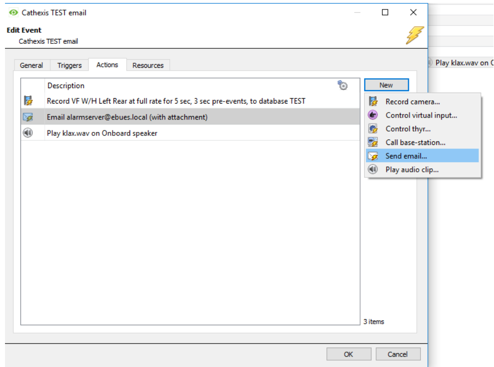
Abbildung 14: Konfiguration von Cathexis-Bildquellen für den Versand von E-Mails (Schritt 2)
